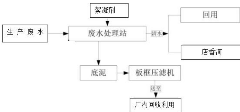
生产废水处理工艺流程图
