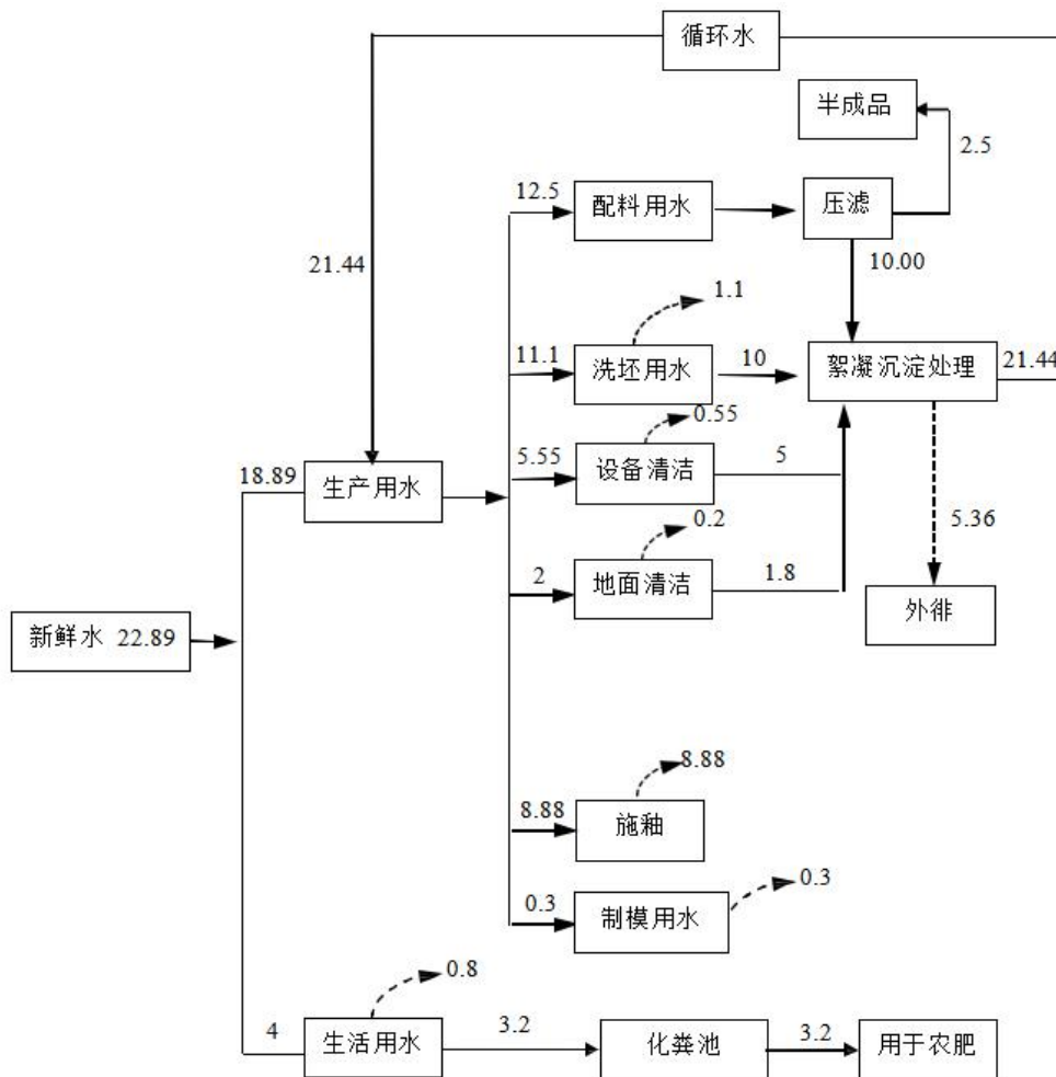
图3-1 项目水平衡图 t/d
