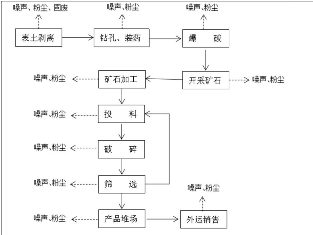
图 4.1-1 矿石开采、加工过程工艺流程及产污节点图
