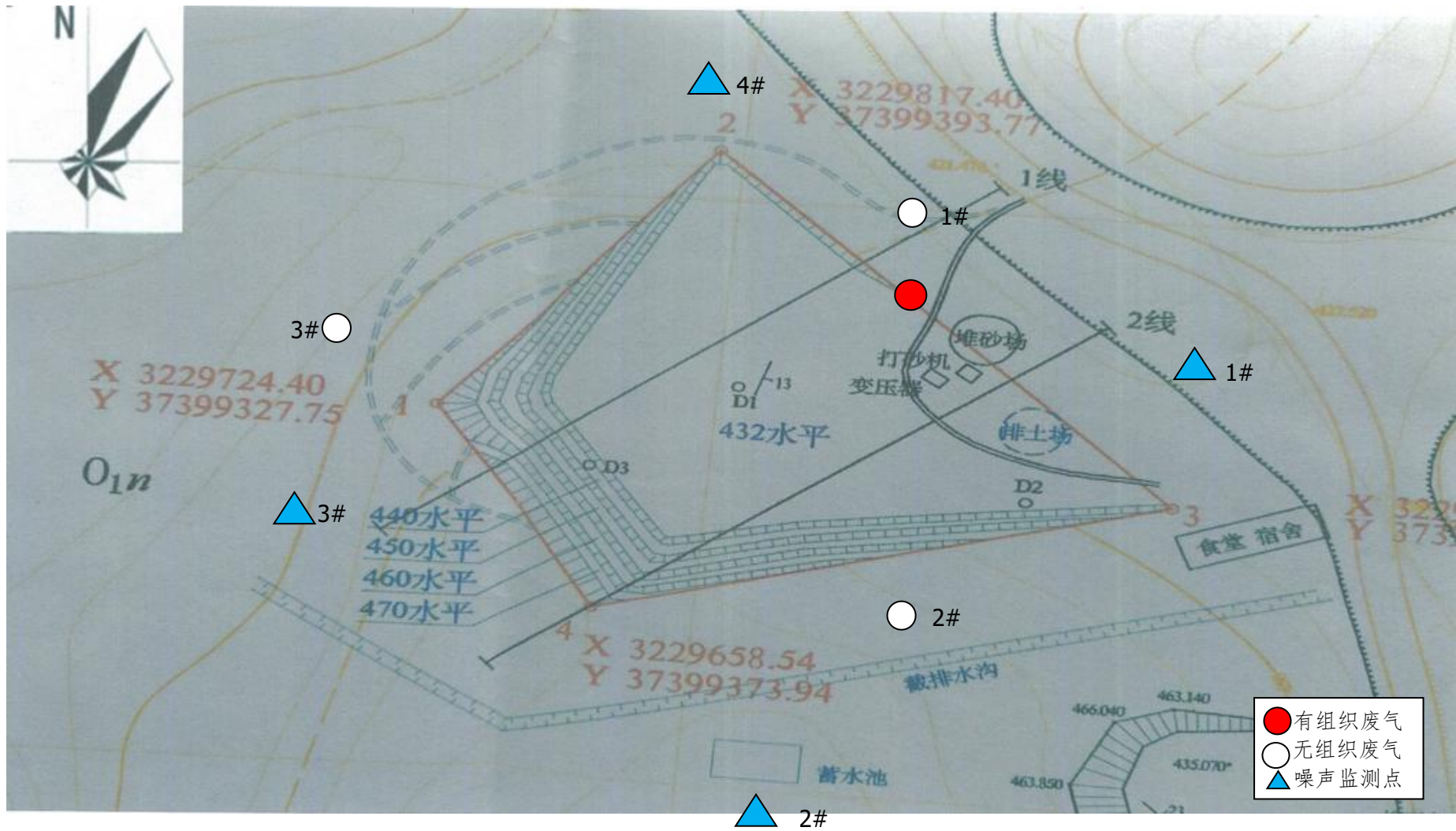
附图 2 项目监测布点及厂区平面布局图
